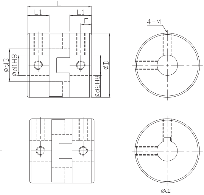
FAMJLK(key way Ød1 side) FAMJRK (key way Ød2 side) FAMJWK (key way Ød1 and Ød2 side)
