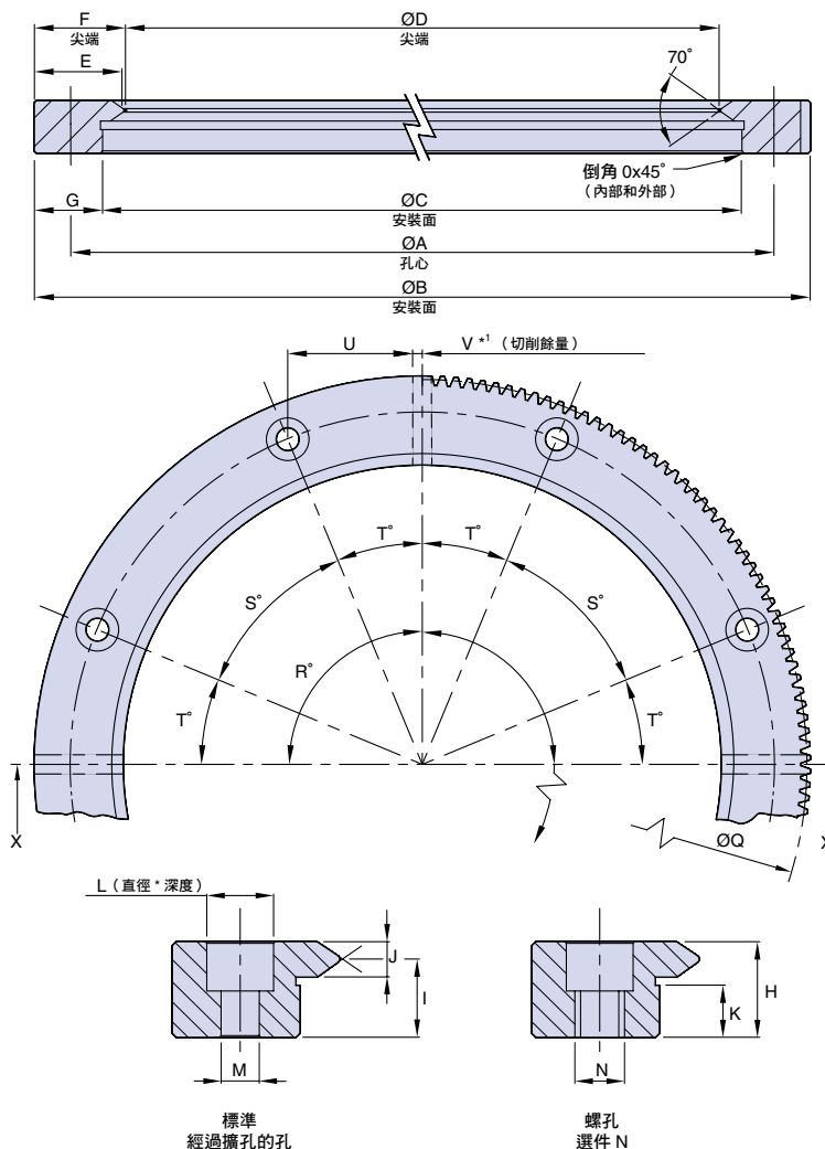
截面 X-X
