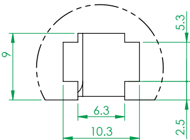
細部放大圖 B 比例 2:1
