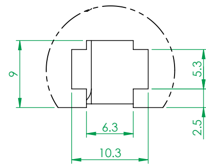
細部放大圖 H 比例 2:1
