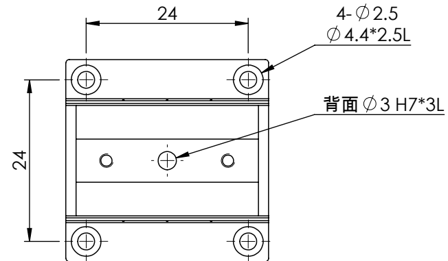
底部安裝孔尺寸
