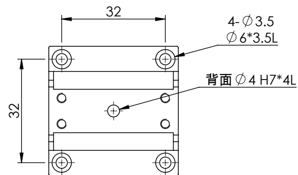
底部安裝孔尺寸
