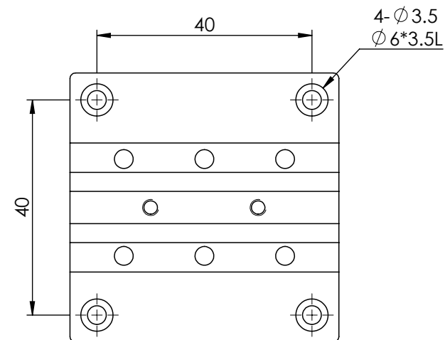
MX(Y)50-A-18系列 底座安裝孔尺寸
