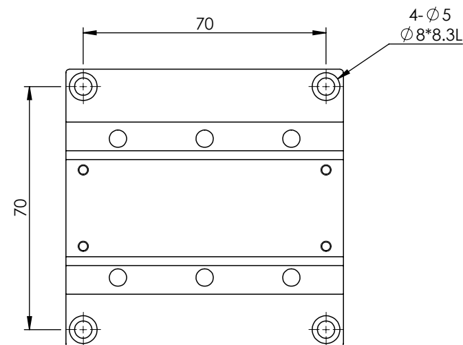
MX(Y)80-A-系列 底座安裝孔尺寸
