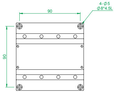
MX(Y)100-A-18系列 底座安裝孔尺寸
