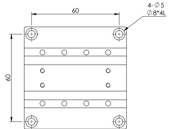
底部安裝孔尺寸
