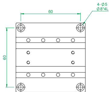
MX(Y)70-A-18系列 底座安裝孔尺寸
