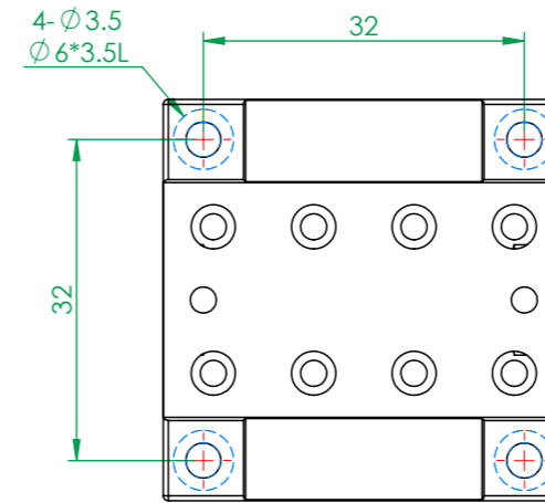
MX(Y)40-A系列 底座安裝孔尺寸
