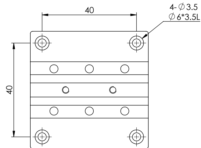
MX(Y)50-A系列 底座安裝孔尺寸
