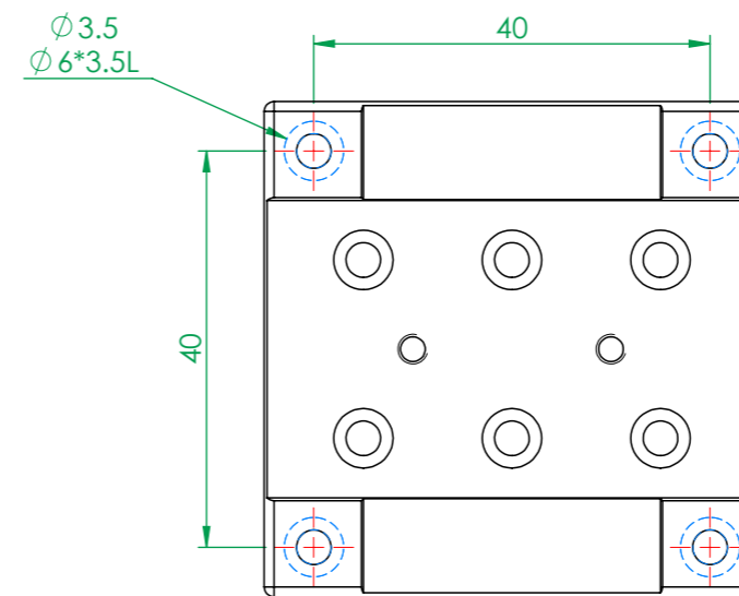
MX(Y)50-A系列 底座安裝孔尺寸
