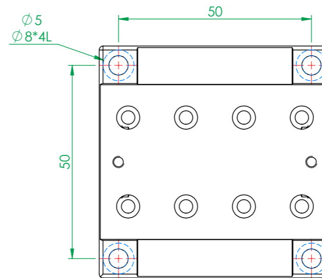
MX(Y)60-A系列 底座安裝孔尺寸
