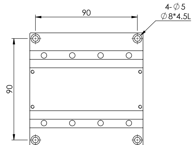
底部安裝孔尺寸
