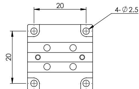
底部安裝孔尺寸
