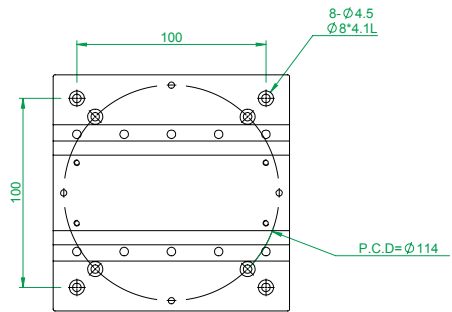
MX(Y)L125-A系列 底座安裝孔尺寸
