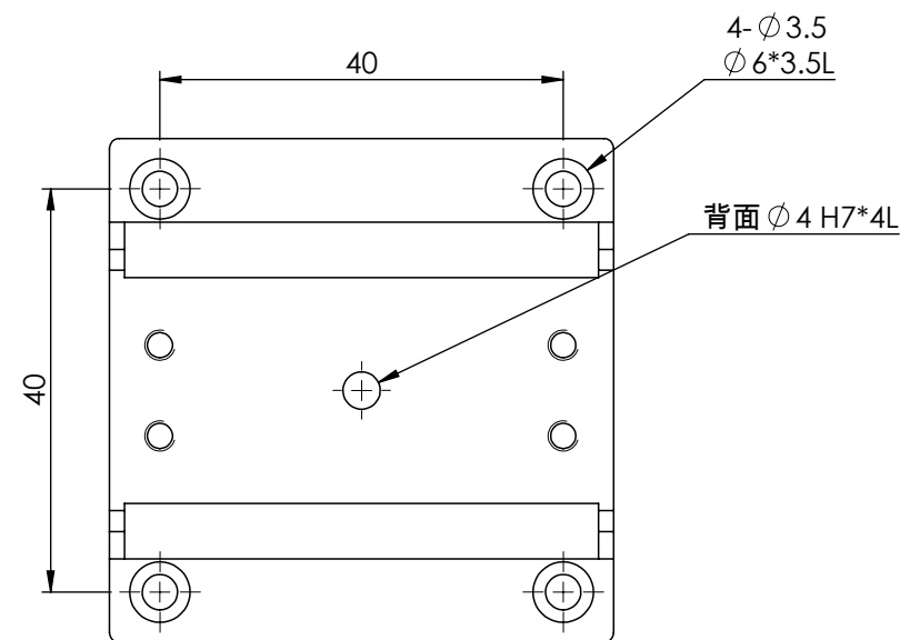
底部安裝孔尺寸
