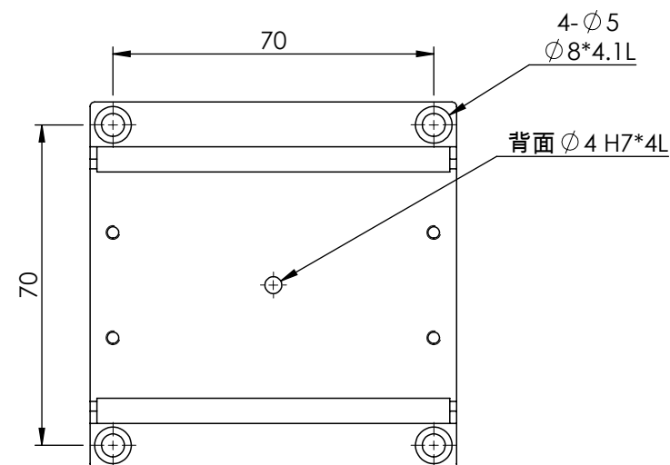
MX(Y)80-S-系列 底座安裝孔尺寸
