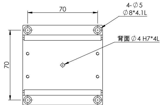
底部安裝孔尺寸
