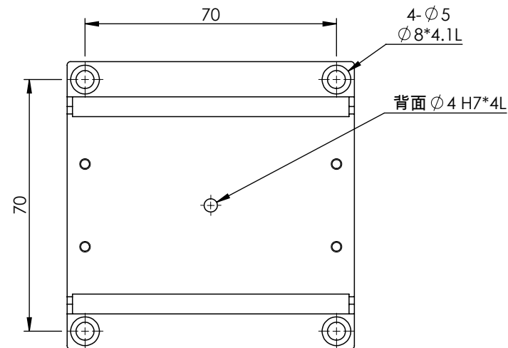
底部安裝孔尺寸
